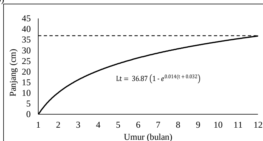
Gambar 3. Kurva pertumbuhan ikan layang berdasarkan persamaan Ford Walford
