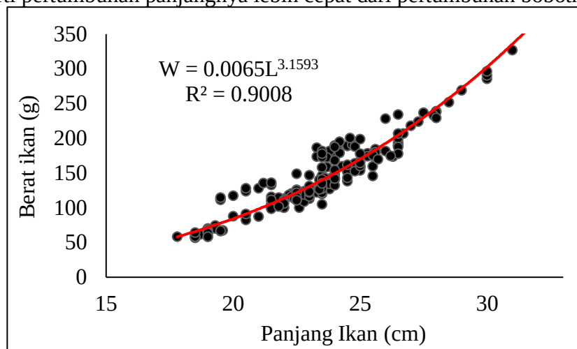
Gambar 4. Kurva hubungan panjang bobot ikan layang
