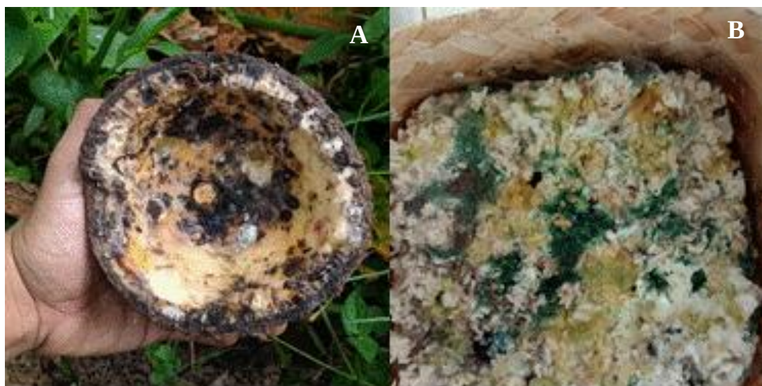
Gambar 1. Hasil eksplorasi jamur antagonis menggunakan media kelapa (A) dan media nasi (B).
