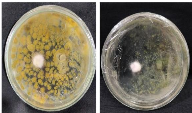
Gambar 4. Uji antagonis jamur Aspergillus sp. (A) dan Trichoderma sp. (B) yang menghambat pertumbuhan jamur patogen Fusarium sp.
