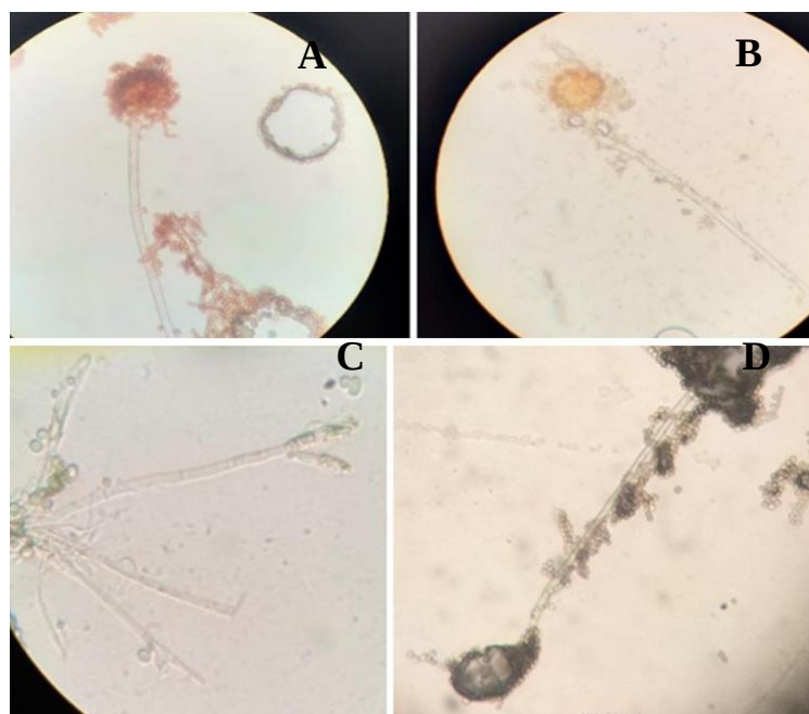
Gambar 3. Hasil identifikasi mikroskopis, jamur warna coklat, jamur warna hijau muda adalah Aspergillus sp, (c) jamur warna hijau tua adalah Trichoderma sp., (d) jamur warna hitam adalah Aspergillus sp.
