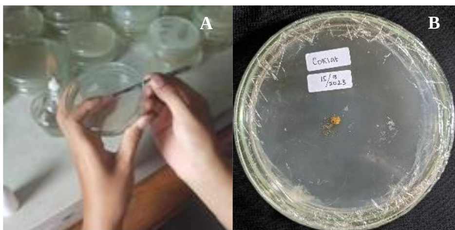
Gambar 2. Inokulasi jamur antagonis hasil eksplorasi menggunakan media PDA. Inokulasi isolat jamur (A) dan hasil inokulasi (B).
