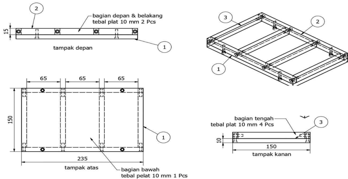
Gambar 5. Cetakan Model A
