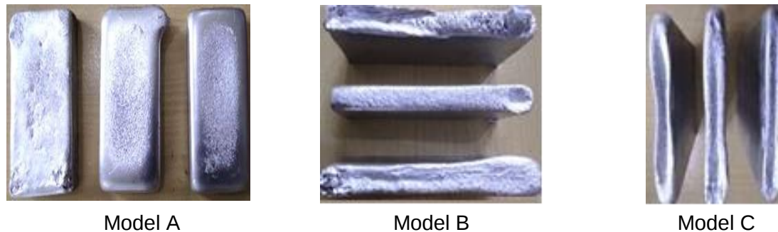
Gambar 10. Hasil cetakan peleburan logam alumunium
