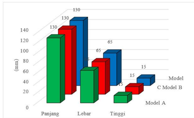
Gambar 12. Dimensi hasil cetakan peleburan logam alumunium
