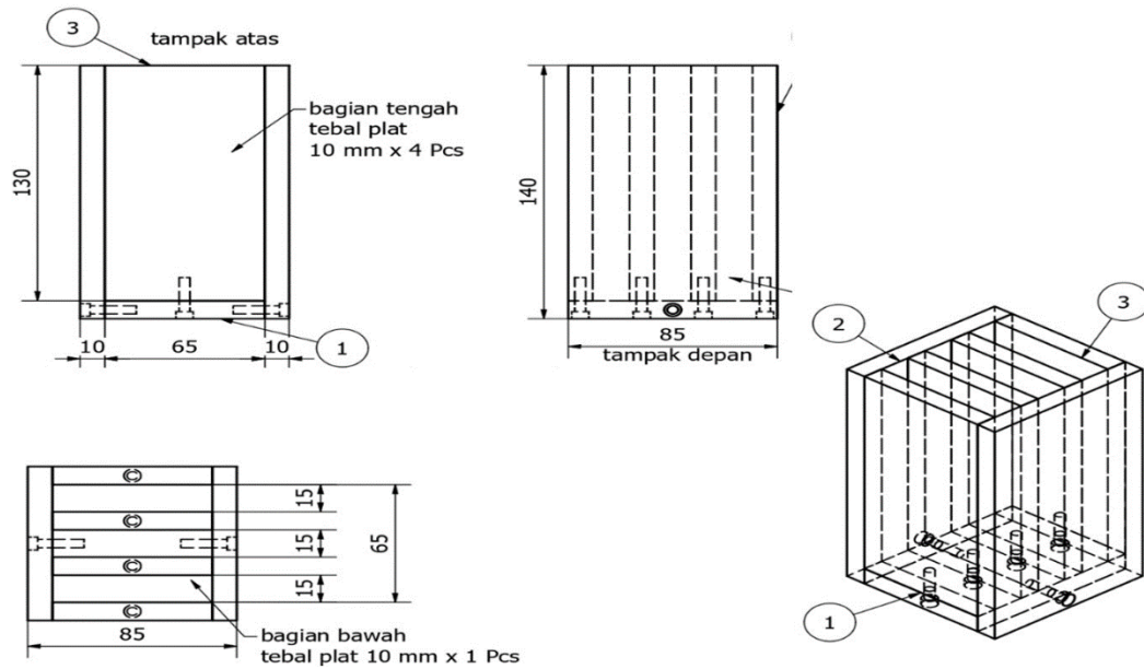
Gambar 7. Cetakan Model C
