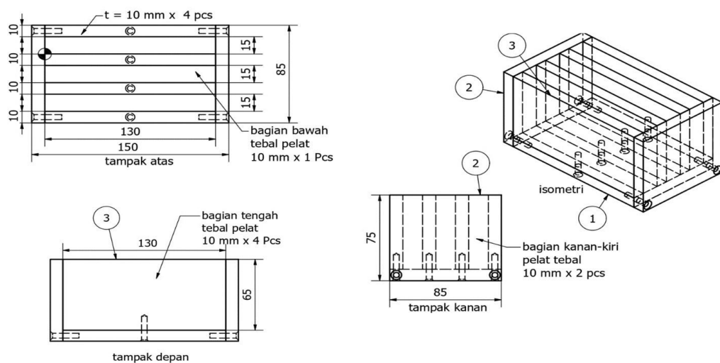
Gambar 6. Cetakan model B
