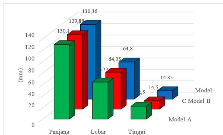
Gambar 11. Dimensi model cetakan peleburan pogam alumunium
